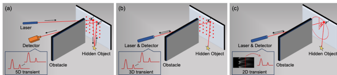
図 1. NLOS イメージングにおける二次元スキャン (a, b) および円形スキャン(c)
