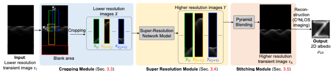
図 2. 超解像を活用した円形スキャンに基づく NLOS イメージングフレームワーク
