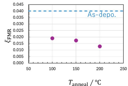
図 5 Si/Al 傾斜材料のみの熱処理した試料のスピントルク効率の熱処理温度依存性
