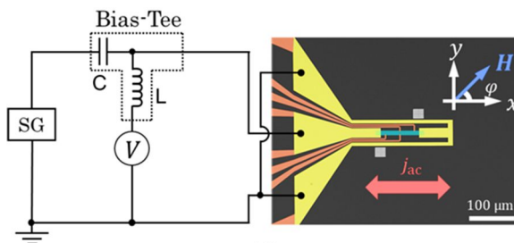
図2 ST-FMR法の測定系概略図
