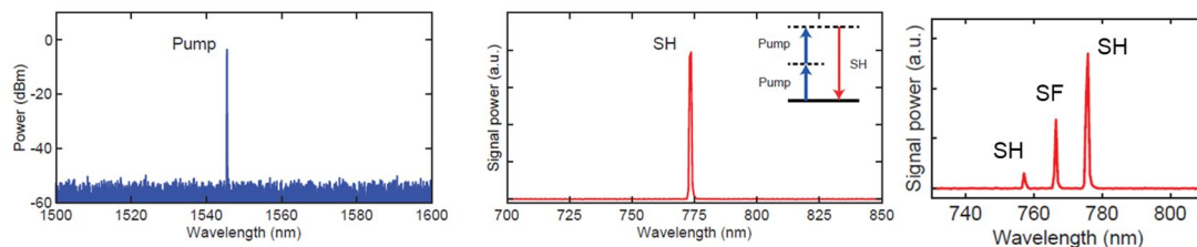
図 3：励起光スペクトルと観測した第二次高調波の光スペクトル。二波長励起時には、第二次高調波発生と和周波発生が同時に発生している。
