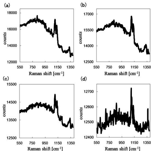
図 4 蛍光除去による S/N の改善: 検出時間はそれぞれ(a) 350 \mu\text{s} (b) 200 \mu\text{s} (c) 100 \mu\text{s} (d) 30 ns
