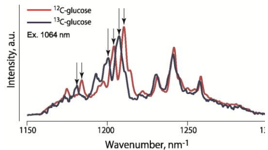
図 5 安定同位体グルコースのラマンスペクトル
