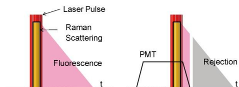
図 2 時間分解蛍光除去法
