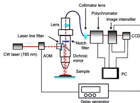
図 1 近赤外高速ゲートラマン分光装置略図
