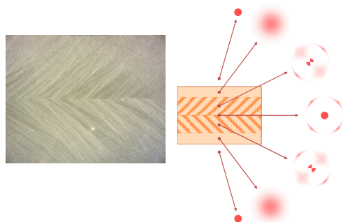
図2 基板上に配向した二クロム酸カリウムのねじれ結晶集積体によって散乱されたレーザ光のスポットパターン
