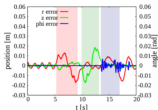
図 12 初期状態（移動前）での作業モード時の動作応答
