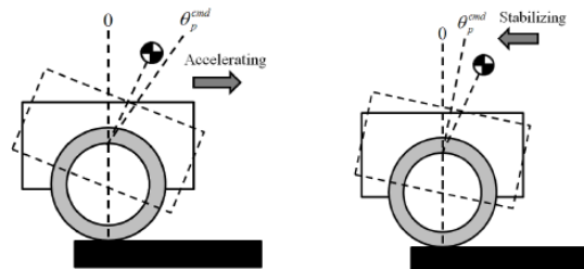
図3 安定制御のみ（左）、安定制御＋リパルシブコンプライアンス制御器（右）
