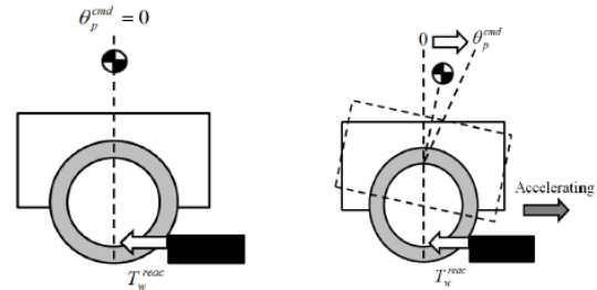
図2 安定制御のみ（左）、安定制御＋リパルシブコンプライアンス制御器（右）
