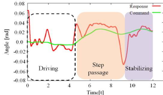
図8 電動車椅子の姿勢応答 (可変ゲイン型リパルシブ制御器)
