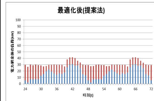
図 3 最適化後の電力網全体の負荷状況
