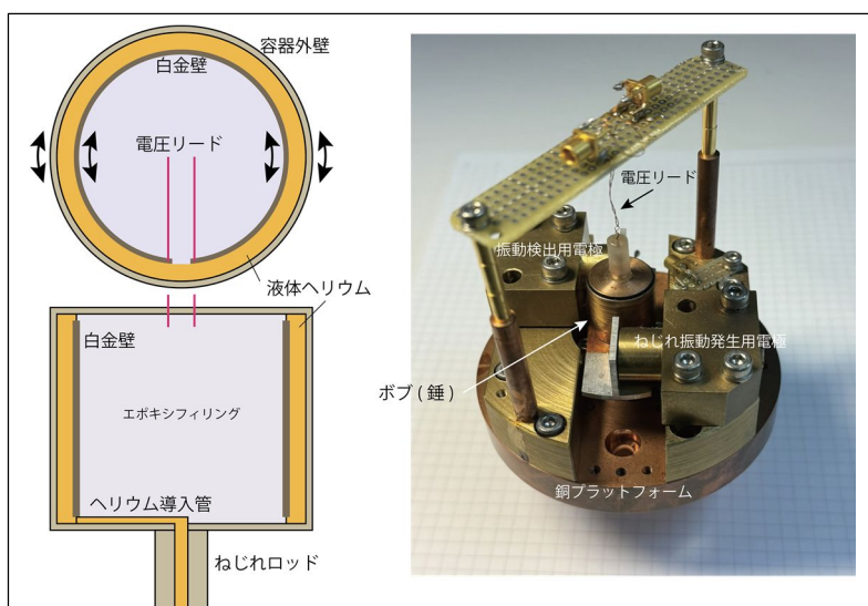
図2: 振動流(スピン流)誘起ねじれ振動子。(左)ねじれ振動子の断面概略図。金属(BeCu)容器に液体 ^3\text{He} が入る円環空間を設ける。内側の壁を白金膜で覆い、ねじれ振動により誘起される両端の電位差を測定する。(右)実際の装置の外観写真。中央にねじれ振動子ボブがあり、2 対の平行平板電極で静電的にねじれ振動を駆動検出する。
