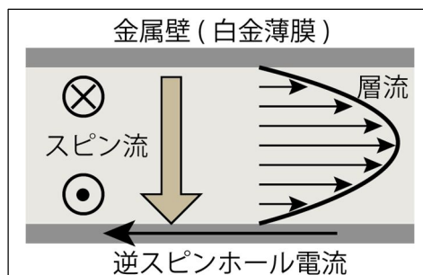
図1: 本研究の概念図。白金薄膜で壁面をコートしたパイプや平行平板中に液体 ^3\text{He} を流すと、速度勾配により生じる渦度が核スピン流(●の向きがスピンの向きに対応)に変換される。白金へのスピン流のしみ出しにより生じた逆スピンホール電流を観測してスピン流の検出を行う。
