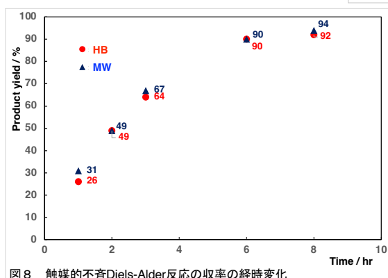
図8 触媒的不斉Diels-Alder反応の収率の経時変化
