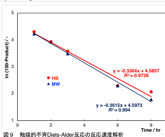
図9 触媒的不斉Diels-Alder反応の反応速度解析
