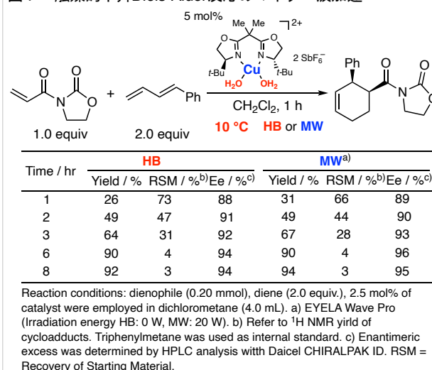
図7 触媒的不斉Diels-Alder反応のマイクロ波加速
