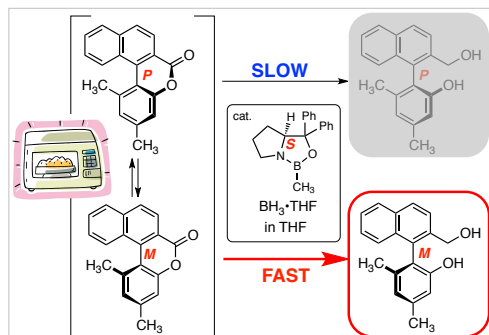
図1 マイクロ波加速のメカニズム
