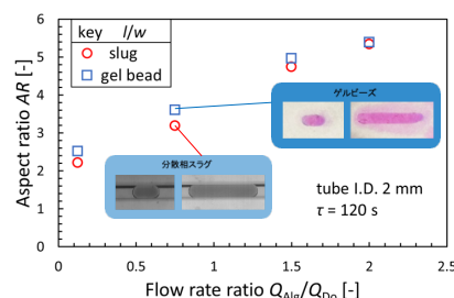
図 4. アルギン酸カルシウムゲルビーズ製造
