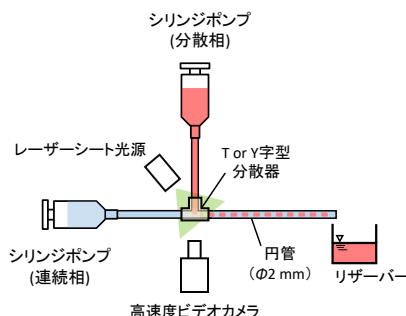
図 1. T 字あるいは Y 字合流によるスラグ流の生成
