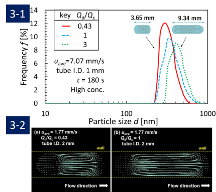
図 3. 分散相スラグでのシリカ生成
