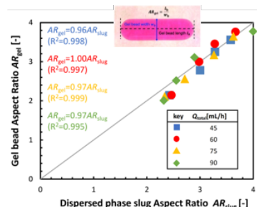
図 5. ゼラチンゲルビーズ製造
