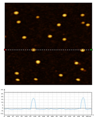
図3. 支持電解質をテトラブチルアンモニウムテトラフルオロボレート、溶媒をDMF、添加剤を水酸化セシウムとした電気化学反応後の \text{FePS}_3 の AFM イメージング
