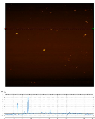
図2. 支持電解質をテトラブチルアンモニウムテトラフルオロボレート、溶媒をDMFとした電気化学反応後の \text{FePS}_3 の AFM イメージング
