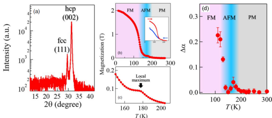
図 5 基板加熱 (623 K) によりスパッタ成膜した Dy 薄膜の (a) X 線回折プロファイル、(b)、(c) 磁化の温度依存性、および (d) スピンポンピング効果の温度依存性
