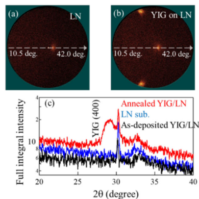
図 3 (a) LN 基板、および (b) LN 基板上に成長した YIG 膜について観察した X 線回折の極点図、(c) X 線回線強度の角度依存性
