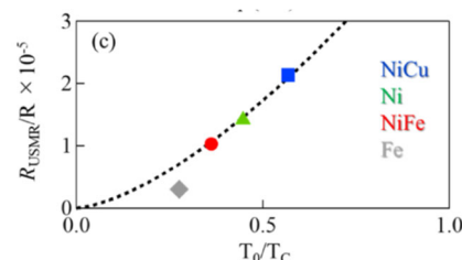
図 2 FM/Pt 2 層膜における USMR 効果のキュリー温度依存性
