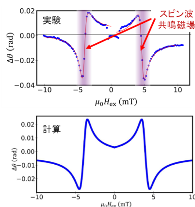
図 1 磁気回転効果による表面弾性波の EdH 位相シフト：(上)実験(下)理論
