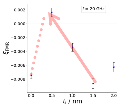
図 4 Ti/W 傾斜材料のスピントルク効率 \xi_{\text{FMR}} の傾斜幅 t_1 依存性
