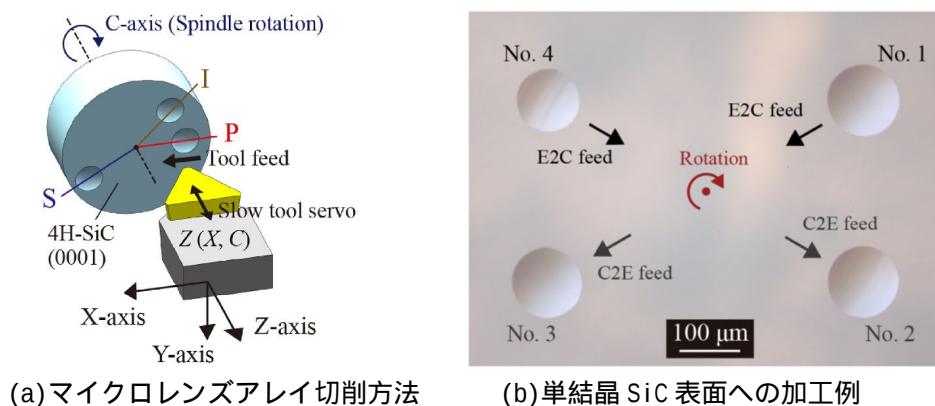
図 1 STS によるマイクロレンズアレイ金型の切削加工
