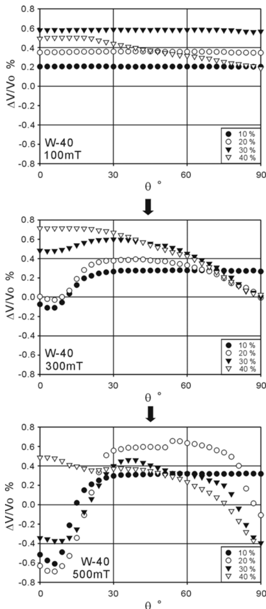
図3 微粒子濃度の音速異方性への影響
