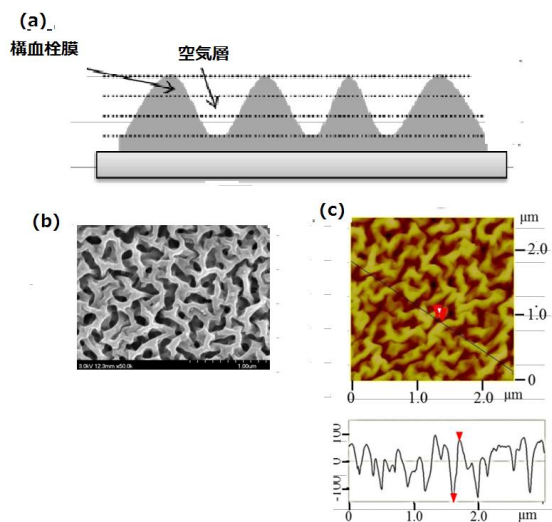
図4 反射防止効果を有する抗血栓薄膜の構造 (a) 反射防止効果を有する抗血栓薄膜の表面構造と屈折率の関係。(薄膜の表面に近い程、空気層を多く含むため、屈折率が傾斜的に減少する。) (b) 反射防止効果を有する抗の電子顕微鏡像 (抗血栓膜の表面に空孔部位が多数見られ、最外部は低密度な楔型構造であることがわかる。) (c) 反射防止効果を有する抗血栓薄膜の表面形状の解析(100~200nm 周期で空気層を持つ楔型構造であることがわかる。)
