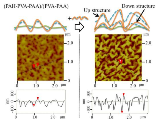
図6 PAH-PAA-PVA 膜表面構造(左)、PAH-PAA-PVA に PAA-PVA を積層した表面構造(右)
