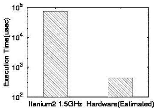
図 6 MUSCL の実行時間の比較
