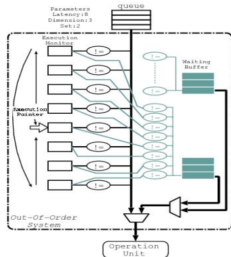
図5 Out-of-Order 機構の構成
