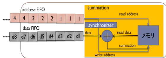
図4 面積分計算のFPGA実装の一部 この処理ではアドレスが指定するメモリのエントリからデータを読み出し、外部からの入力と足し合わせて、同じエントリに書き戻す。読み出しから書き戻すまで数クロックかかる。処理中のデータを要求する場合、そのデータが処理されメモリに格納されるまで
