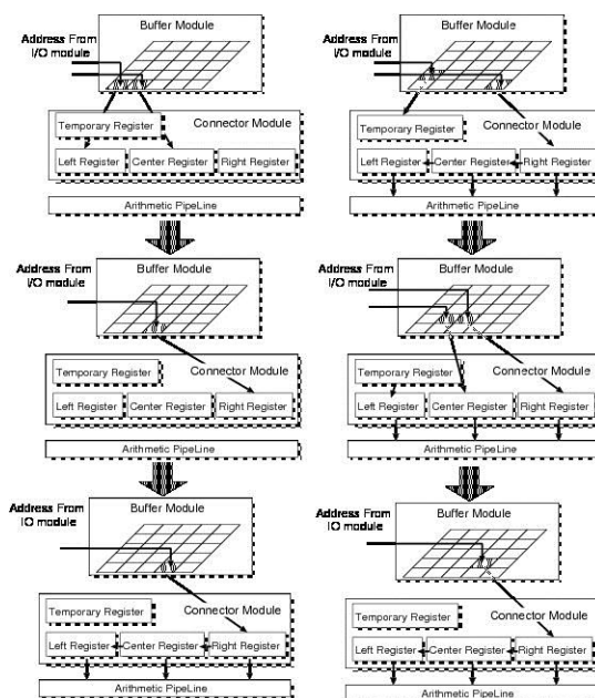
図 2 MUSCL のアクセスコントローラ
