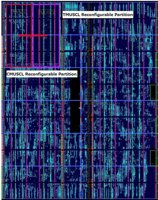
図3 Virtex-3上のレイアウト
