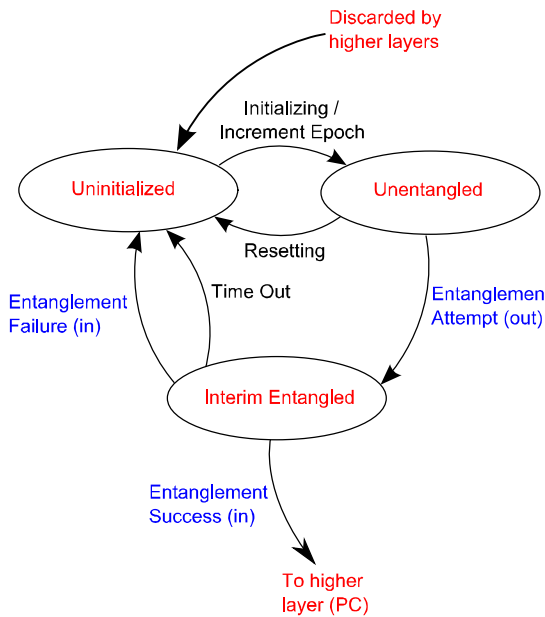
図 4 Entanglement Control Protocol 有限状態機械 (送信側) 青い字は転送するメッセージである。
