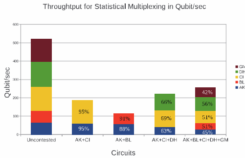
図 6 Statistical multiplexing における、実験通信パターンと達成された帯域
