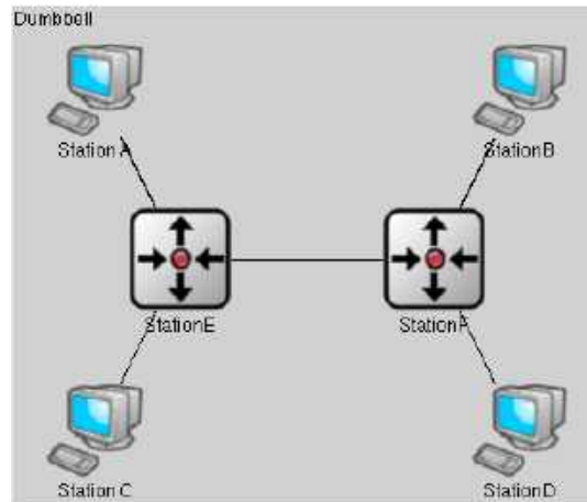
図 1 Sapphyre 量子リピーターネットワークシミュレーターのネットワークトポロジーの画面
