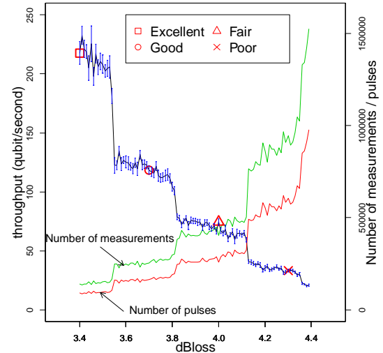
図 7 Qubus 型のリピーターの一ホップのシミュレーション
