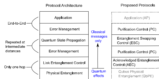
図 3 階層型のプロトコルスタック：概念
