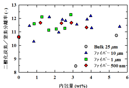
図 4 PMPS / PDMS コンポジットの二酸化炭素 / 窒素分離係数の変化。
