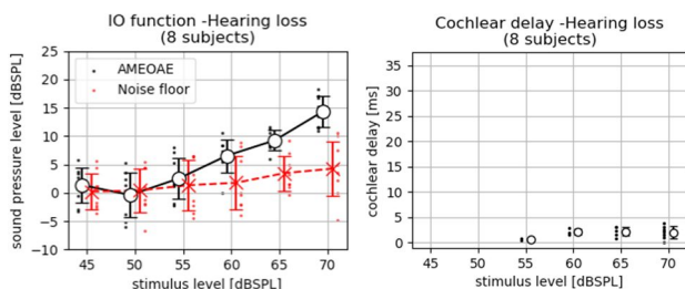
図 3：難聴者 8 名における AMEOAE の入出力特性と推定された蝸牛遅延
