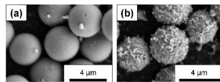
図 4 (a) 球状チタニア粒子および (b) 球状 \text{CaTiO}_3:\text{Pr}^{3+} 粒子の SEM 写真
