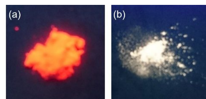
図 3 (a) \text{CaTiO}_3:\text{Pr}^{3+} (302 nm 照射) および (b) \text{CaZrO}_3:\text{Pr}^{3+} 粉末試料 (254 nm 照射) の発光の様子
