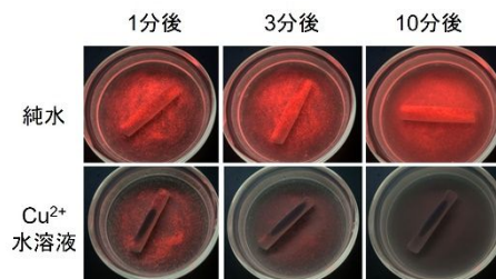
図 2 紫外線 (254 nm) を照射しながら純水および \text{Cu}^{2+} 水溶液に分散させた MOF 由来 \text{Gd}_2\text{O}_3:\text{Eu}^{3+} 粉末試料の 1、3 および 10 分後の様子
