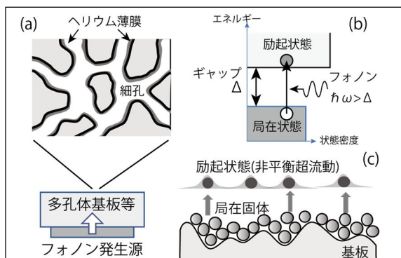
図 2 非平衡超流動の実現方法。(a)吸着基板に接したフォノン発生源より、ヘリウム薄膜にフォノンを照射する。(b)(c)フォノンエネルギー \hbar\omega がエネルギーギャップ \Delta を越えれば、局在状態から広がった励起状態にヘリウムが励起されて超流動状態に加わる。
