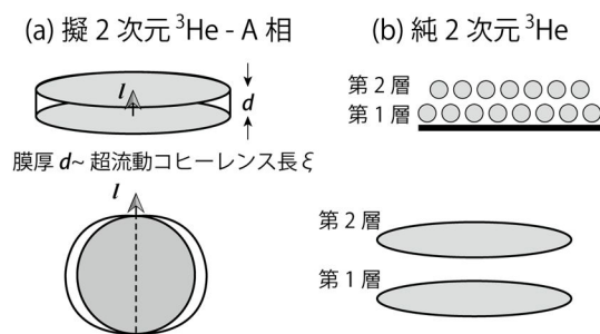
図 3 擬 2 次元と純 2 次元 ^3\text{He} の違い。(a)擬 2 次元(A 相を例に取る)はコヒーレンス長の数倍(約 100nm)の膜厚で、フェルミ面上にギャップを持つ。(b)純 2 次元 ^3\text{He} は、層ごとにフェルミ円盤を形成し、ギャップは円盤の縁にある。
