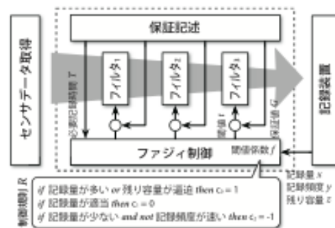
図 2 記憶容量予約機構概要図
