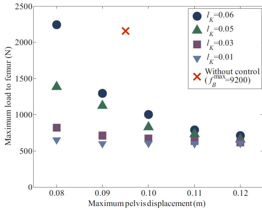
図2 最大ラップベルト荷重 6000 N の場合の腰変位拘束と大腿骨荷重最大値の関係 (×:最大ラップベルト荷重 9200 N、膝部初期クリアランス 0.06 m)
