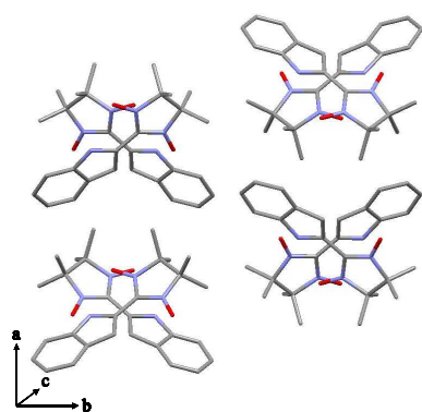
図1 1の結晶構造(c軸投影図)
