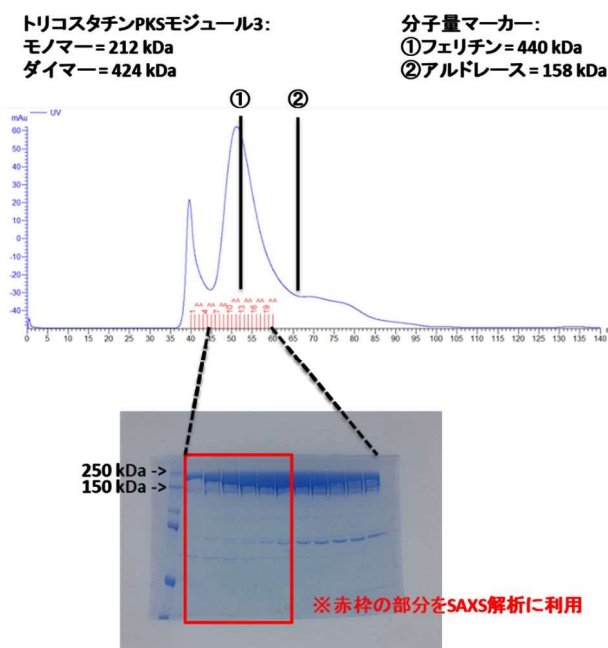
図3 トリコスタチンPKSモジュール3のゲルろ過精製
