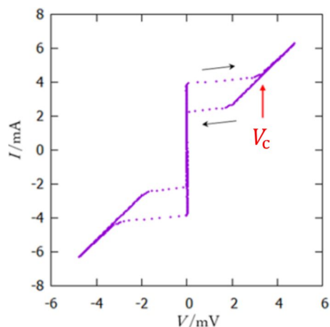
図 2: 作成した Nb-(Al)-AlO x -Nb トンネル素子の電流電圧特性。測定温度は 3.5K。電圧状態への遷移時の臨界電圧 V_c より、超伝導エネルギーギャップ 2\Delta が得られる。理想的な接合では電圧減少時に V_c 以下で電流が流れない(大きなヒステリシスが生じる)が、本接合ではリーク電流が生じていることがわかる。
