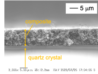
図 1 作製した合剤塗布電極の断面 SEM 像.
