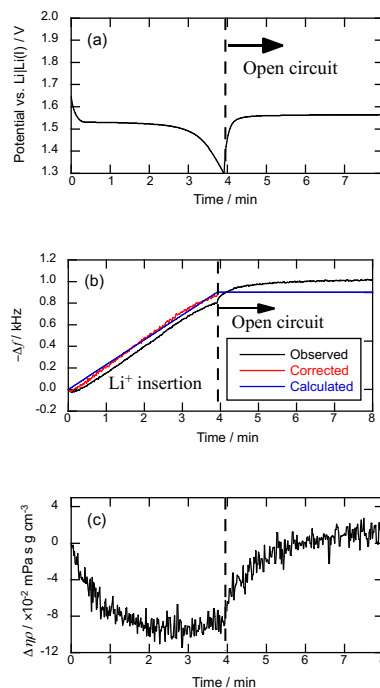
図 4 LiTFS/EC+DMC 中における LTO 合剤塗布電極の定電流 \text{Li}^+ 挿入時の EQCM 応答 (a) 電位, (b) 周波数変化および (c) 局所 \eta\rho 変化。
