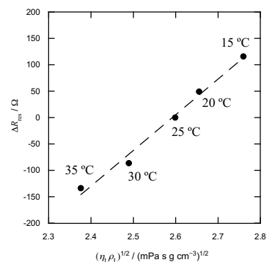
図 3 異なる温度での電解液の \eta\rho 値と R_{\text{res}} の関係.
