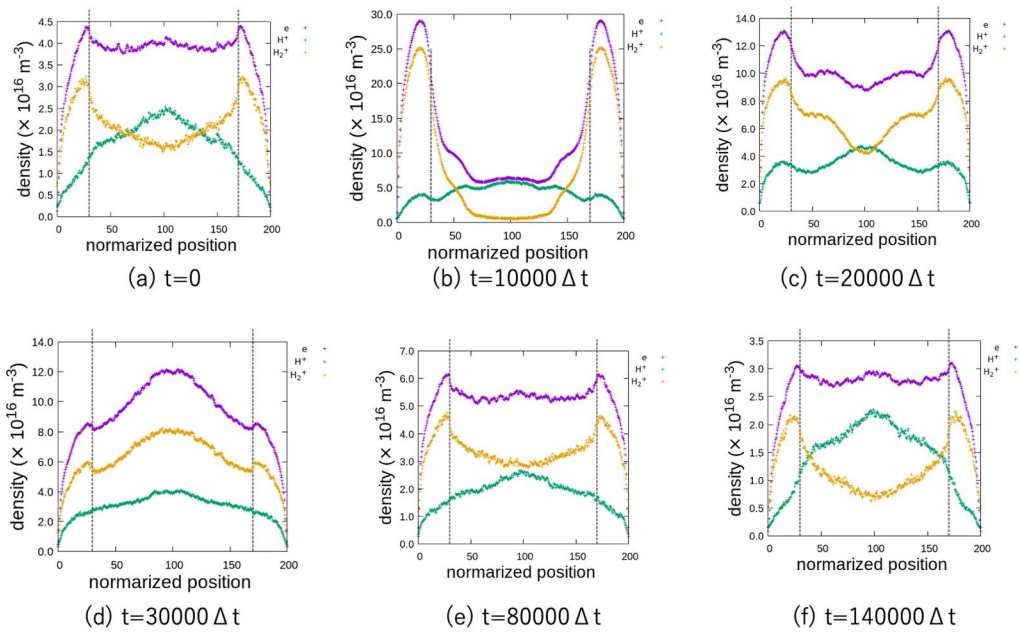
Fig.3 プラズマ密度分布の熱パルス入射による時間変化。 \Delta t はシミュレーションのタイムステップ。
