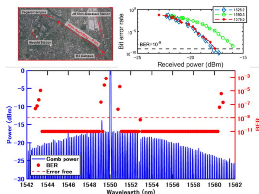
図 7: 市中ファイバを用いてマイクロコムを多波長光源として DWDM 伝送を実証。
