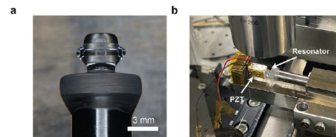
図 3: \text{MgF}_2 共振器の圧力による波長制御の実験系
