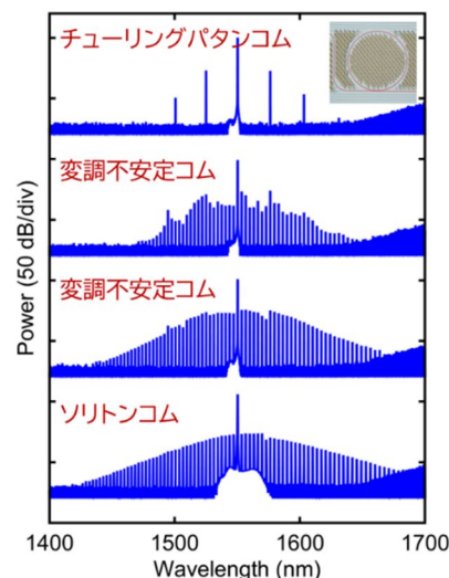
図 6: シリコンナイトライドリングで生成したマイクロコムの比較検討。
