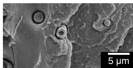
図 15. PEKnF/PSt の破面観察
