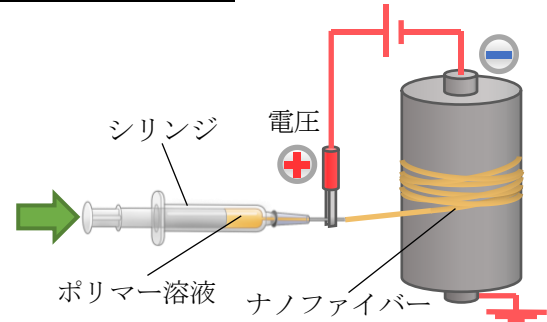
図 2. エレクトロスピンニング法
