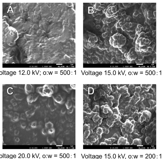
図 2 印加電圧、エマルション比率を変化させたナノ粒子の形状評価
