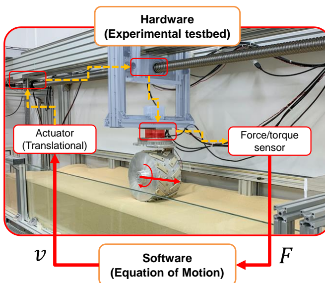
図 1：不整地用 HILS
