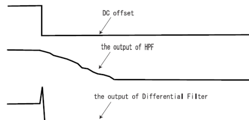
図 3.3 DC オフセットの影響と微分フィルタ
