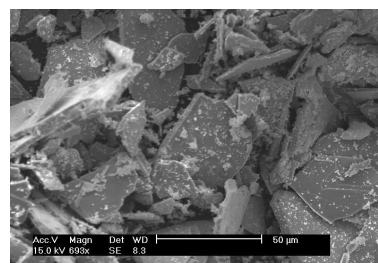
図 1 板状 \text{Ba}_6\text{Ti}_{17}\text{O}_{40} 粒子の形状
