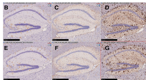
図 4. 5xFAD における グリオシス・神経炎症に対する AQP4 欠損の影響 (A) グリオシス・神経炎症のマーカーの発現を定量的 PCR で測定した。(B-G) 40 週齢の 5xFAD/AQP4 KO (B-D) 及び 5xFAD (E-G) の海馬周辺の矢状断パラフィン包埋切片の A \beta (B, E)、GFAP (C, F) 及び Iba1 (D, G) の染色。
