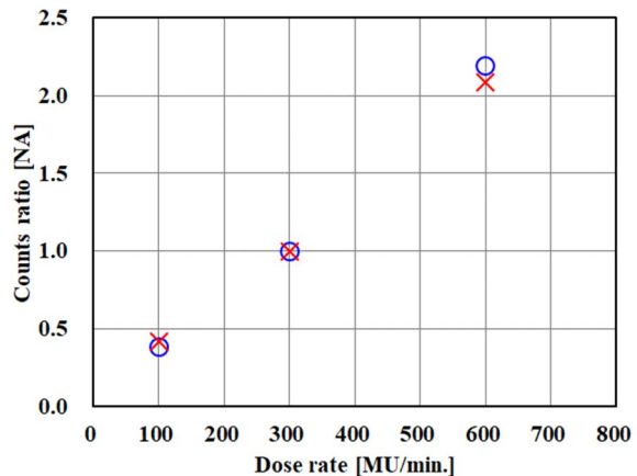
図5 10 MV のエネルギーに対する線量率と計数率の関係(線量率 300 \text{ [MU/min.]} で正規化)。×は計測した全 BG、○は 400-600 keV の範囲に存在する BG。
