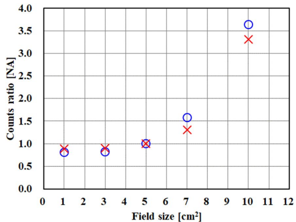
図4 10 MV のエネルギーに対する照射野と計数率の関係(照射野 5.0 \times 5.0 \text{ cm}^2 で正規化)。×は計測した全 BG、○は 400-600 keV の範囲に存在する BG。
