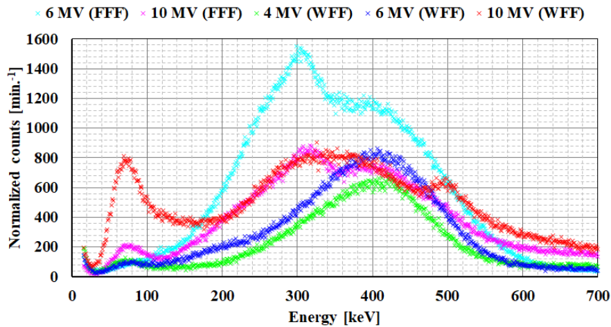
図3 各治療ビームのエネルギーから取得したエネルギースペクトル。照射野 5.0 \times 5.0 \text{ cm}^2 、計数率は各エネルギーの線量率を 250 \text{ MU/min.} に正規化して算出している。
