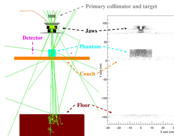
図2 放射線輸送計算の展開例。右図の散布図は、左図のMCSにより検出器に入射した光子の発生位置の計算結果に対応している。
