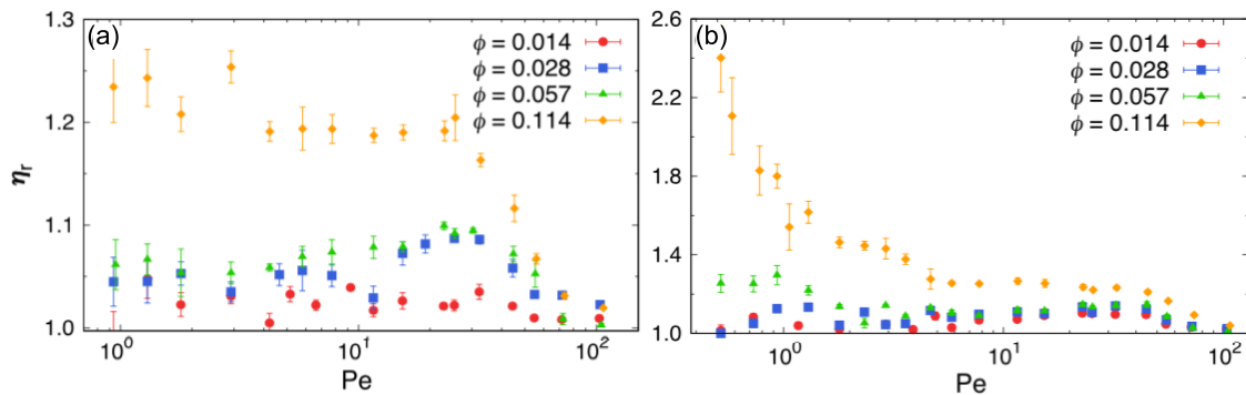
図4 相対粘度とペクレ数の関係 (a) 疎水割合: 少, (b) 疎水割合: 多
