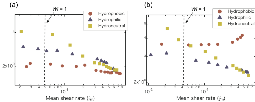
図1 粘度と平均せん断速度の関係 (a)10%, (b)30%
