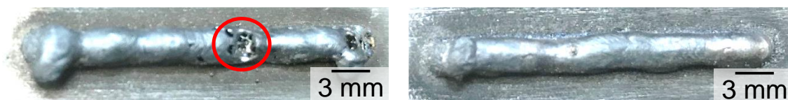
図4 左：テルル無添加の造形物表面 右：テルル 1 wt%添加の造形物表面
