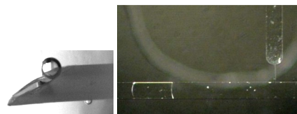
図 6 マイクロチャネル内スラグ(右)と水中への気泡放出(左)
