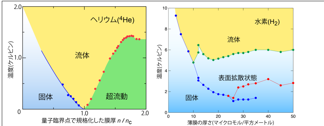
図3: 弾性異常の温度から得られる相図。左が ^4\text{He} 、右が水素薄膜の相図を示す。両者ともに膜の厚さを増やすと固化温度が急激に減少し、ヘリウムは量子臨界点で超流動になる。水素では約1Kまで表面分子の拡散が保持され、過冷却液体状態にある(青点)。
