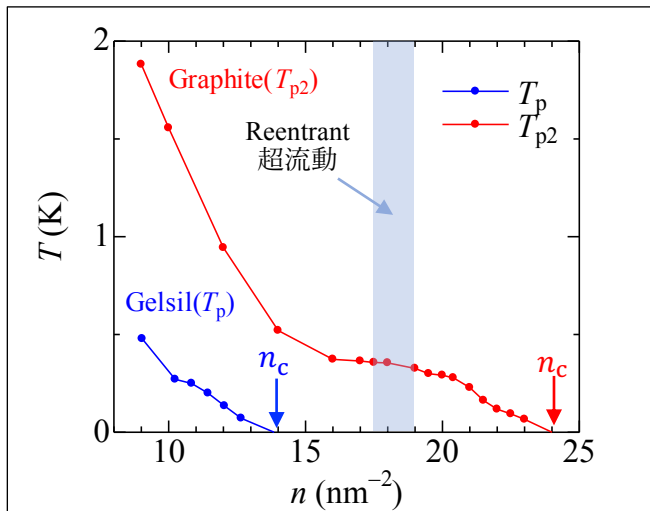
図4: グラファイト上 ^4\text{He} 薄膜における第2の弾性異常温度(散逸ピーク温度) T_{p2} の吸着量依存性(赤色)。15-20 \text{nm}^{-2} でプラトーを持ち、別の実験で示されるリエントラント超流動領域と重なるため、超流動と剛性の共存が示唆される。またガラス基板(Gelsil 多孔ガラス)上での異常温度。
