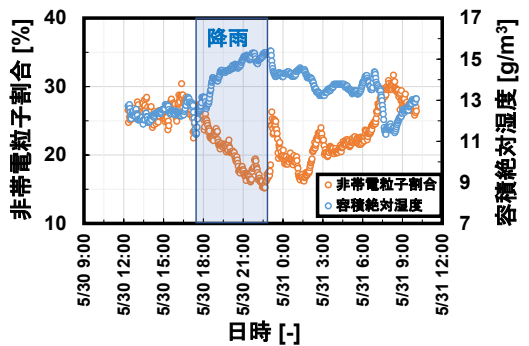
Fig. 3 雨天時の非帯電粒子割合の連続測定 (測定期間：2018/5/30～2018/5/31, 測定地点：横浜市, 対象粒径：0.3-0.5 μm)
