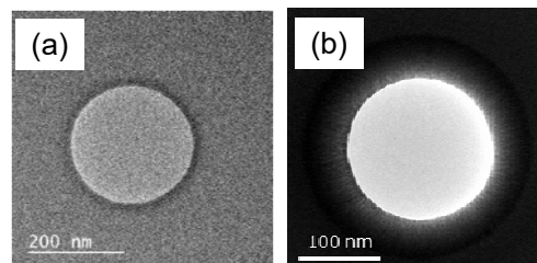
図 7 (a) GST 成膜前と (b) 成膜後のナノポアの TEM 画像
