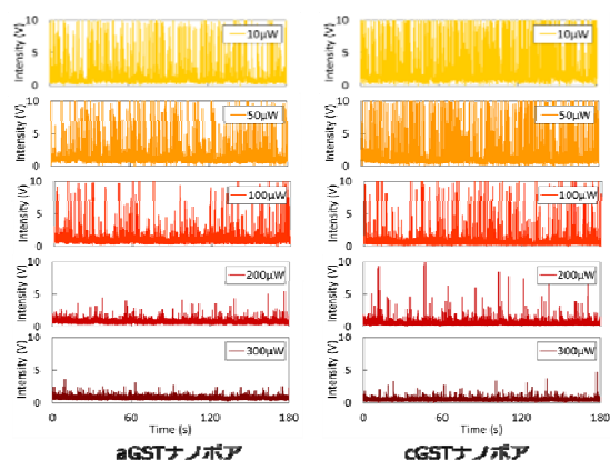
図11 DNA ナノポア通過時の蛍光バースト信号
