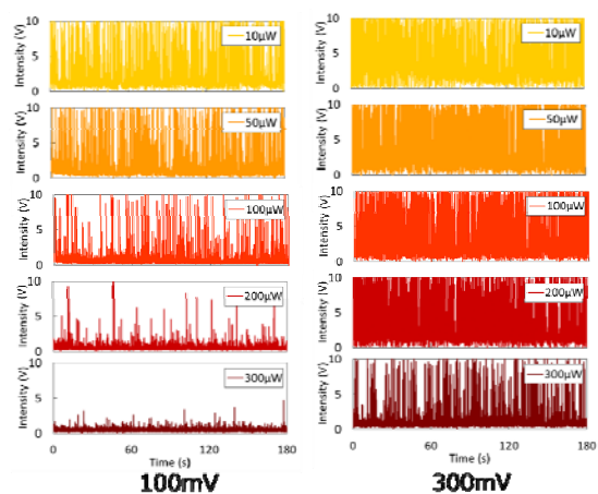
図12 DNA ナノポア通過頻度の印加電圧依存性
