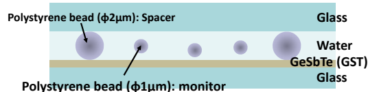
図 4 GeSbTe 光熱効果実証のためのチャンネル構造
