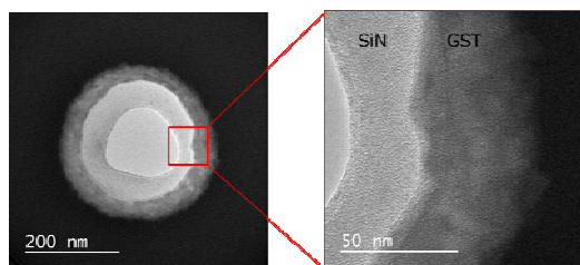
図8 保護膜なし GST ナノポアの計測後の TEM 画像
