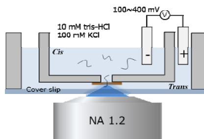
図 1 ナノポア光学検出用チャンパー
