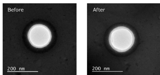
図9 \text{SiO}_2 保護 GST ナノポアの計測前後の TEM 画像
