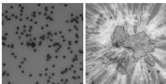
図10 GST 膜上での対流発生を観察結果
