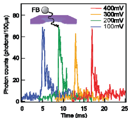
図 5 蛍光ポリスチレンビーズのナノポア通過波形
