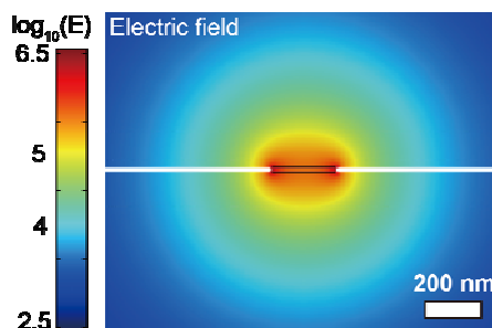
図 2 ナノポア近傍の電界分布
