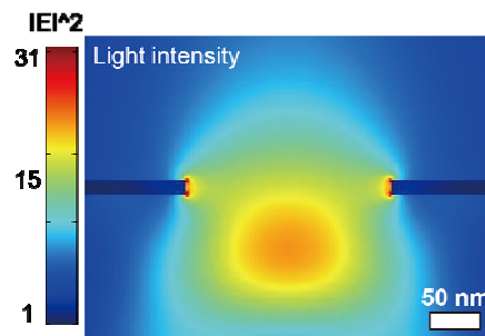
図 3 ナノポア近傍における光強度分布
