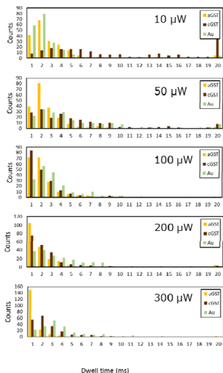
図 13 DNA ナノポア通過時間の励起光強度依存性
