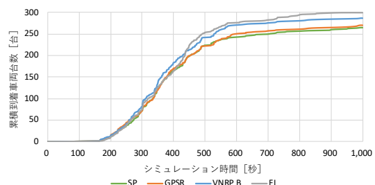
図 10 累積到着車両台数 (N = 300)
