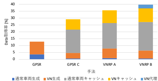
図 9 Data 取得率の比較
