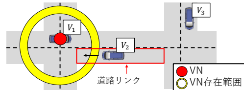
図 2 仮想ノード(VN)とVN存在範囲
