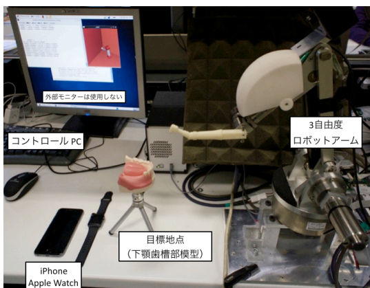
図 5 実験機材
