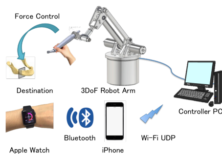
図2 試作機概略図
