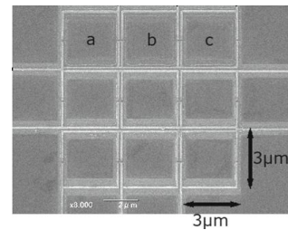
図 2. マイクロ SQUID 配列
