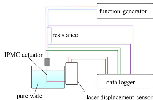
図3：繰返し変形時の電気的特性評価試験
