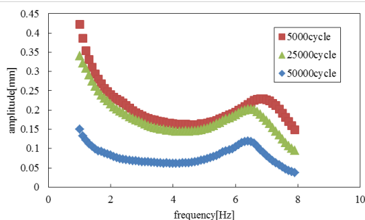
図 4：振幅と周波数の関係
