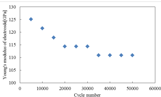
図 5：電極ヤング率とサイクル数の関係
