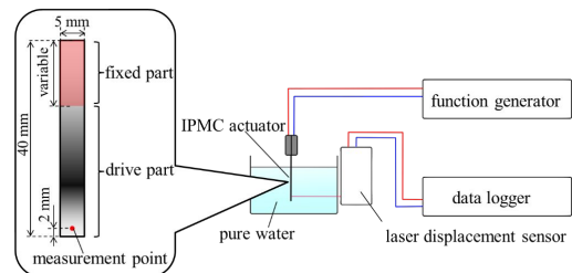
図2：繰返し変形時の機械的特性評価試験
