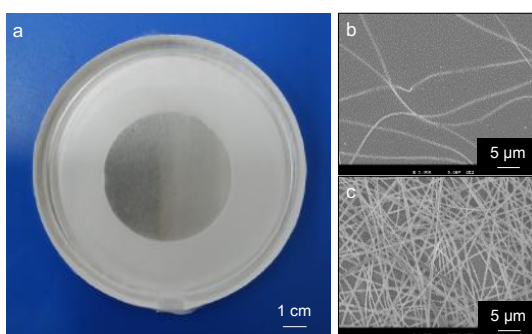
図 8 パターンニングされた PLA ナノファイバシート(a)とその SEM 画像 (b)未処理面、(c)プラズマ処理面
