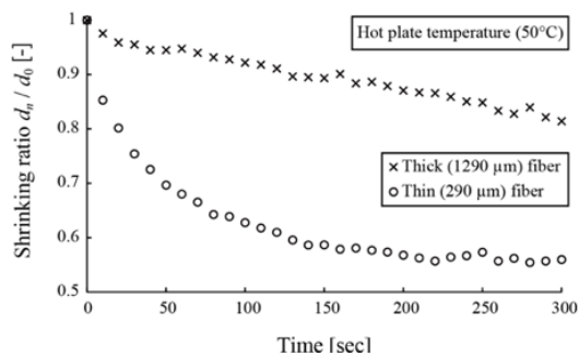
図2 ゲルファイバの時間応答。
