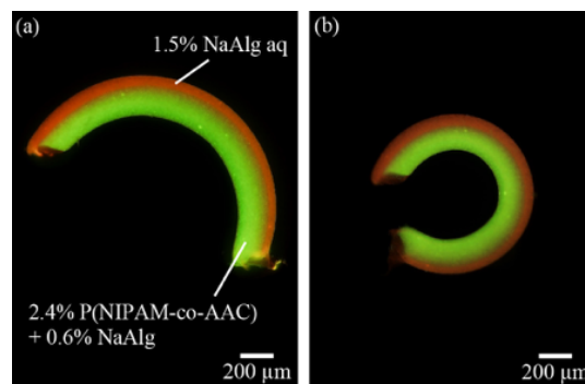
図3 二層ゲルファイバの刺激への応答。(a) 刺激前。(b) 刺激後。
