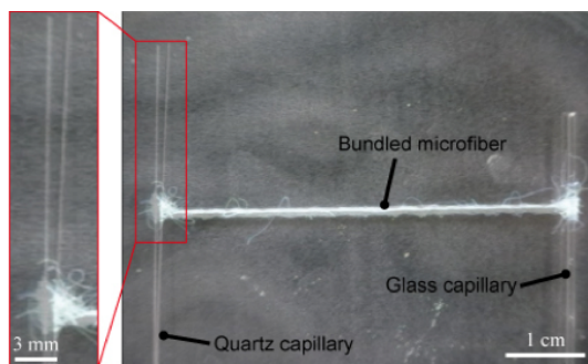
図9 バンドル型ゲルアクチュエータ (上). 収縮力の計測の様子
