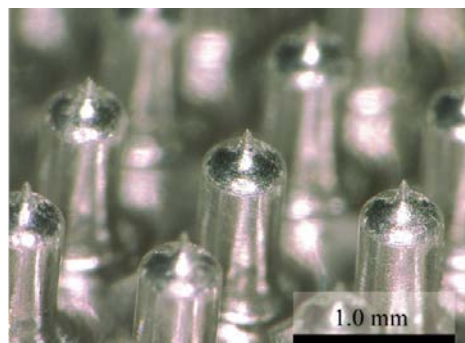
図4. キャンドル型微小針電極
