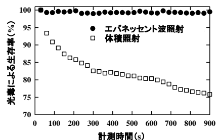
図6 エバネッセント波照射、および体積照射による、HUVEC 細胞の生存率変化。
