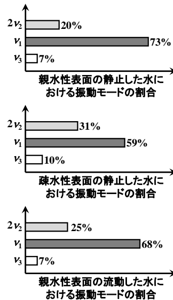
図2 表面性状の違いによる、水分子の振動モードの変化。
