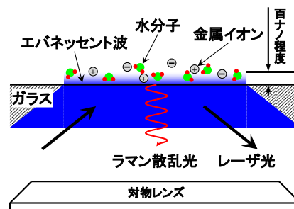
図1 エバネッセント波照射による、界面極近傍に存在する水分子やイオンからの、ラマン散乱光の撮像を行う概念図。
