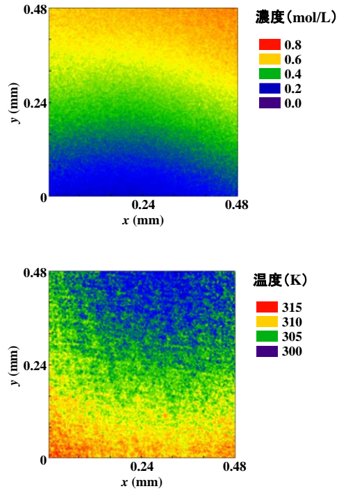
図4 三波長ラマン散乱光イメージング法による、 \text{Na}_2\text{SO}_4 溶液の濃度と温度の時空間分布の同時計測結果。
