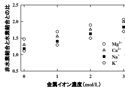
図3 界面極近傍における、金属イオン混入による、水分子の水素結合状態の変化。
