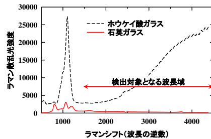
図5 ホウケイ酸ガラスと石英ガラスからのラマン散乱光強度分布。ラマン散乱光イメージング法では、石英ガラスを用いた方が、ノイズが大幅に低減される。
